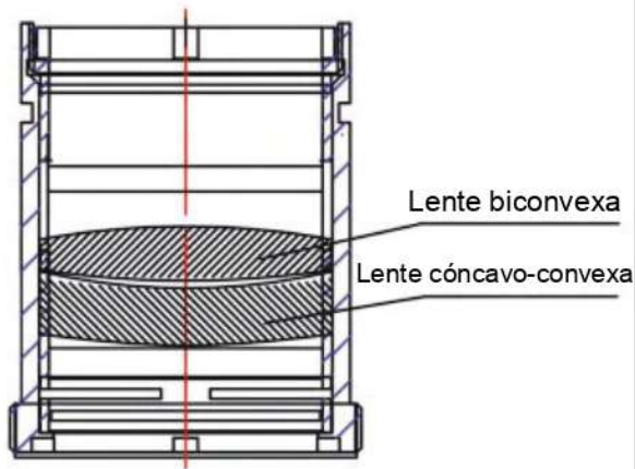
Estructura del lente de enfoque
